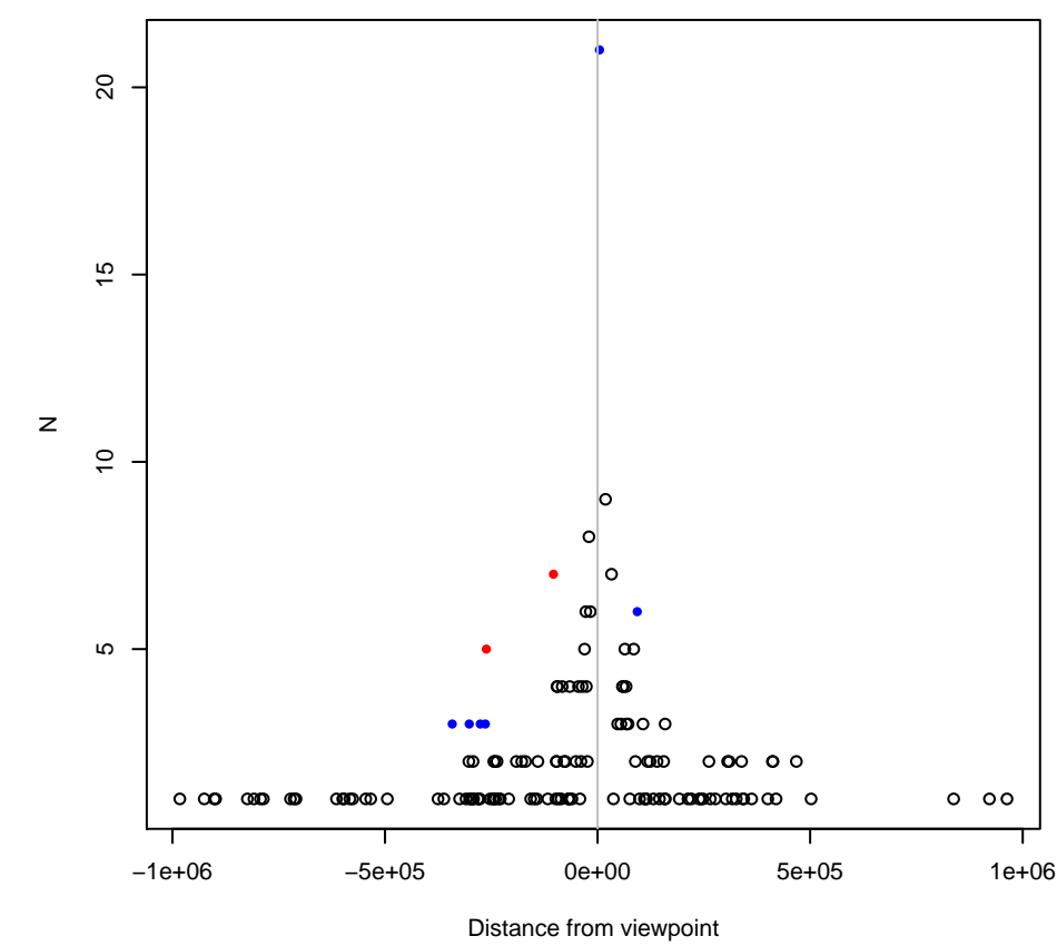
CNOT7;VPS37A (712239)
