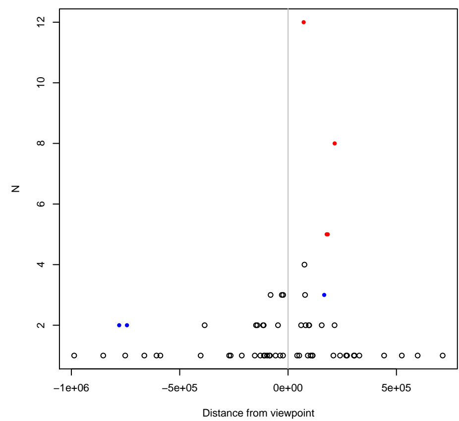
RNU6-623P (292328)
