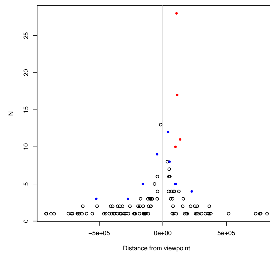
AL589765.1;CELF3;RIIAD1;RP11-98D18.1 (35739)
