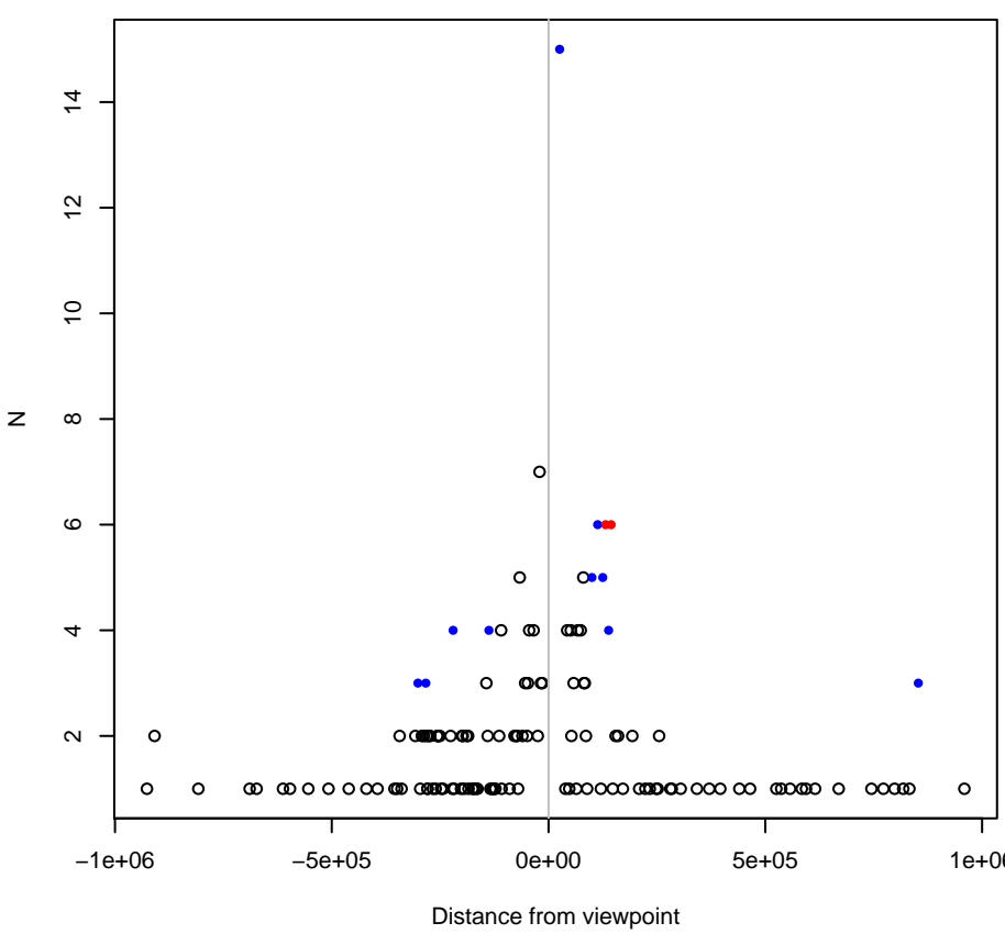
NA (185009)
