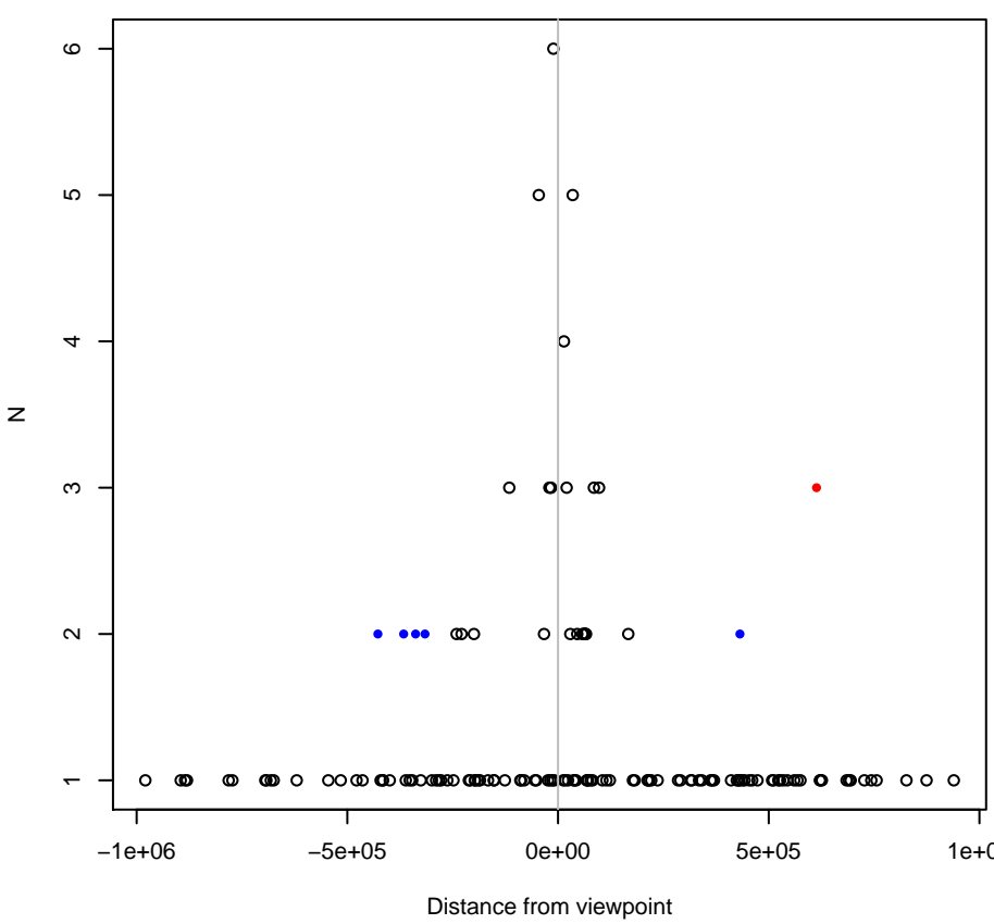
RP3-467L1.4 (1490)
