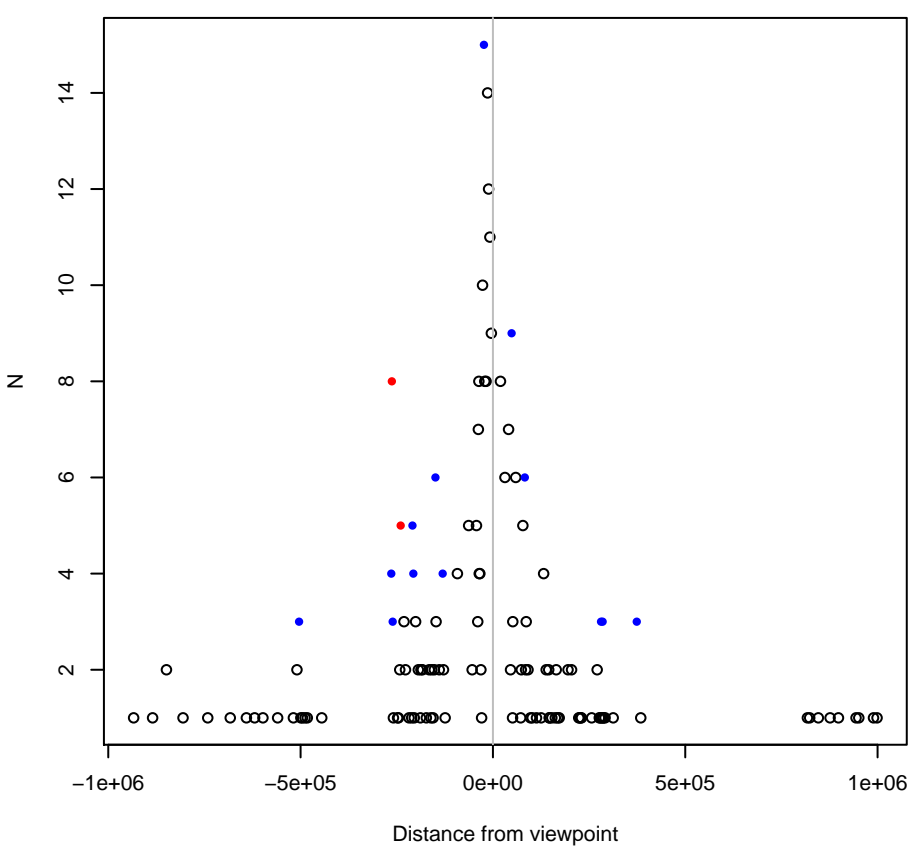
DNAJB8-AS1 (474938)
